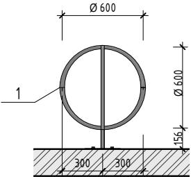
Разрез 2 - 2 (1 : 25)
