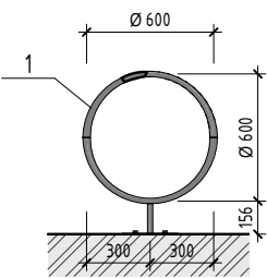
Разрез 3 - 3 (1 : 25)
